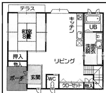
間取り図 1階
